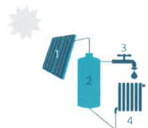
1 Zonnecollector | 2 Opslagvat zonneboiler | 3 Sanitair warm water | 4 mogelijke element voor ruimteverwarming optioneel
